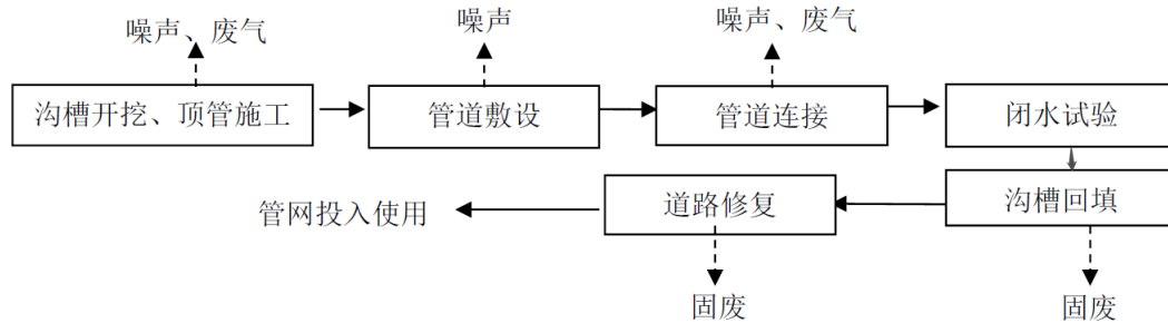
图 3.1-1 管道施工工艺流程及产污环节图
